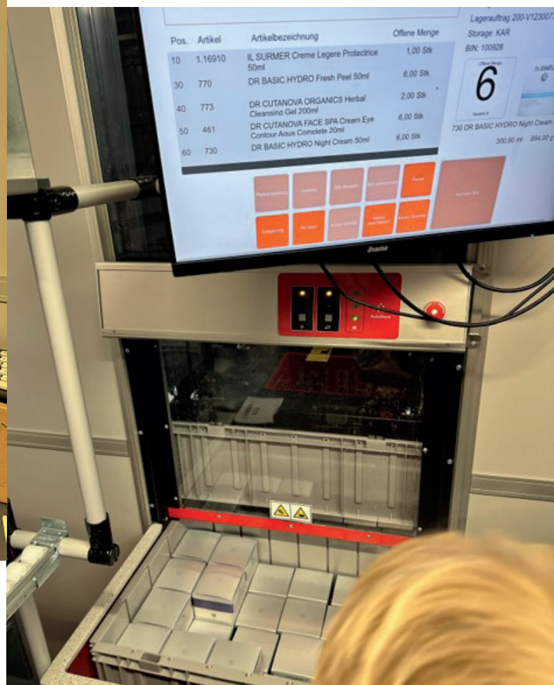
Entnahme der korrekten Menge und Bestätigung auf dem Display
